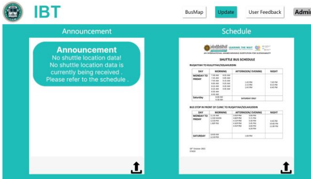
Fig. 15. Update page
