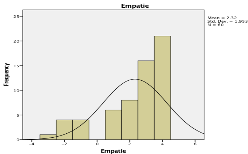
Fig. 4.5 Empathy
