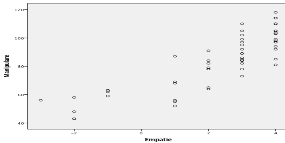
Fig. 4.6 Manipulation – empathy
