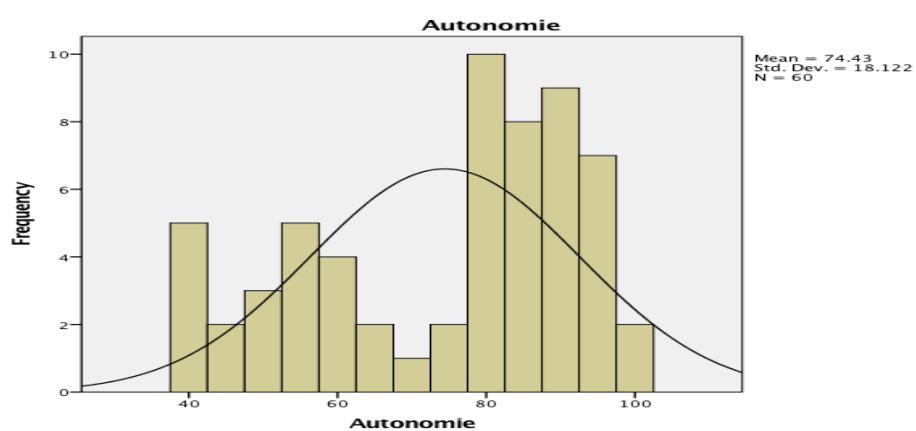
Fig. 4.11 Autonomy
